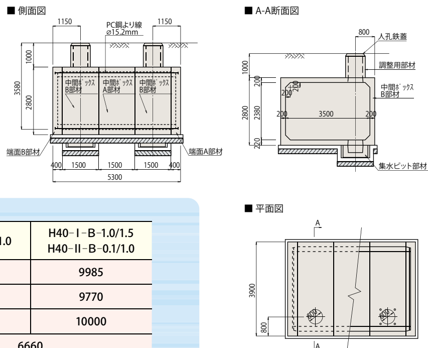
Bタイプ構造図(40㎡)
