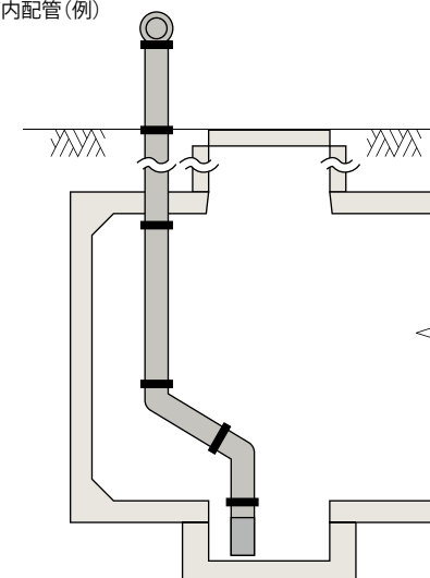
■水槽内配管(例)
