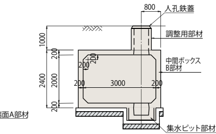
A-A断面図
