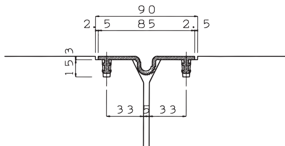
ロングV用ゴムジョイント
