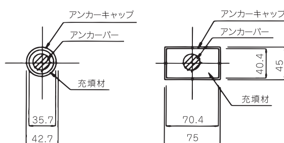
アンカー部詳細図
