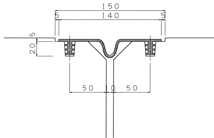
ロングスパンフリューム用ゴムジョイント
