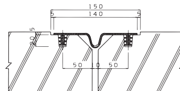
ケース2 DFTゴムジョイント
