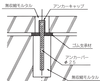
支承部詳細図
