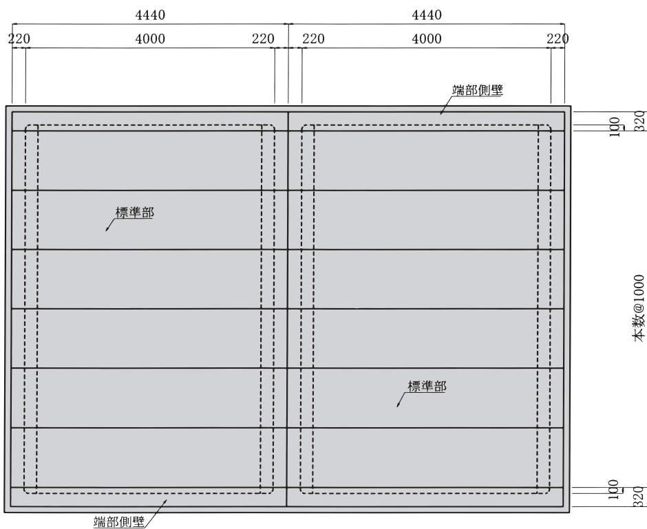
平面図
