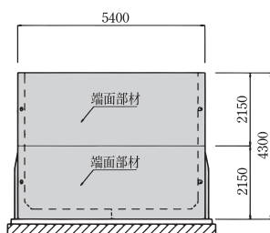
正面図
