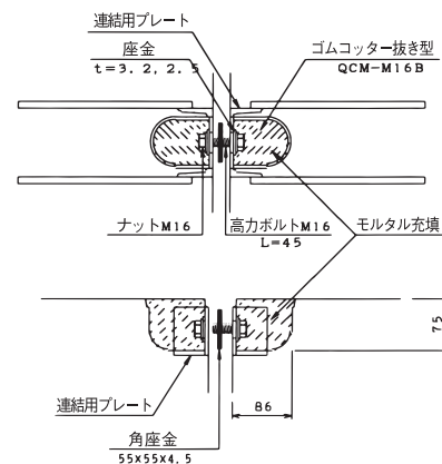
連結部詳細図
