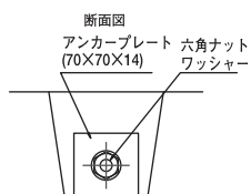
製品連結例 (1)
