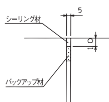
外目地部詳細図
