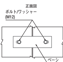
製品連結例 (2)
