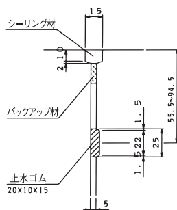
内目地部詳細図
