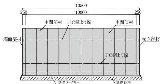
側面図
