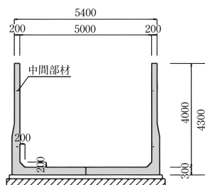
断面図
