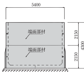
正面図
