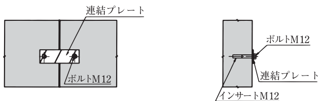
連結部詳細
