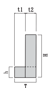
側面図
